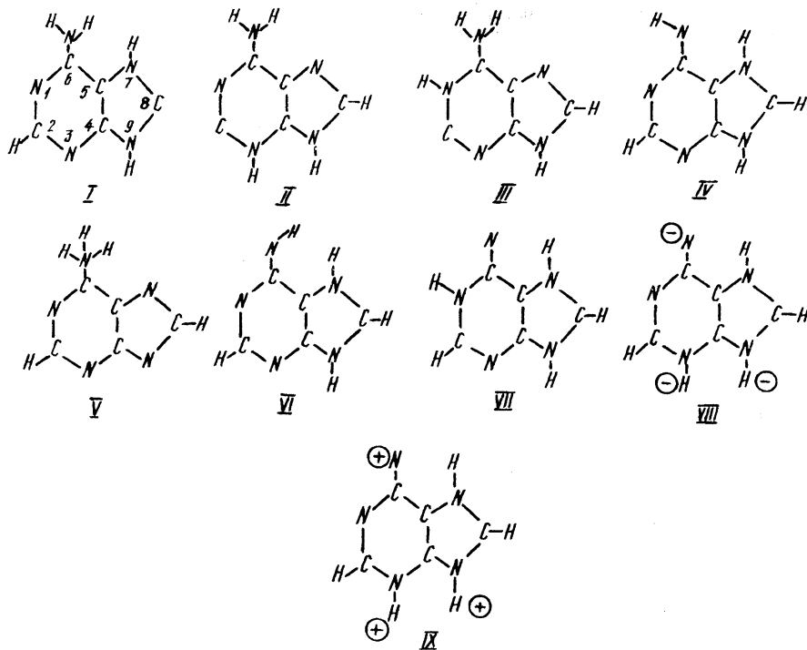
Рис. 1. Сімейство прототропних таутомерів-цвітеріонів аденіну, включаючи три найнижкоенергетичніші ілідні форми I—III. Тут і на рис. 2 знаками «+» і «-» позначено максимальні відхилення атомів від площинності
